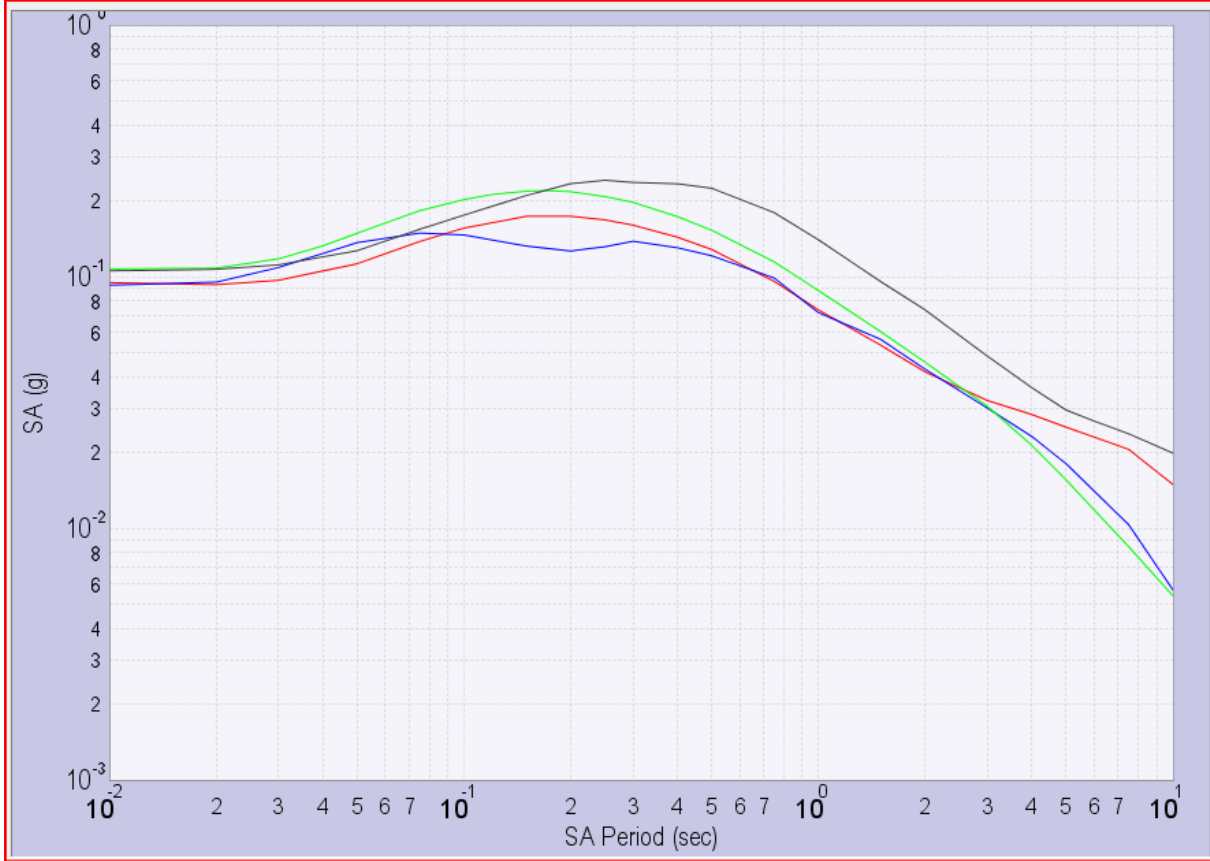
Şekil 3.6: Deterministik %5 Sönümlü Yatay İvme Spektrumu
