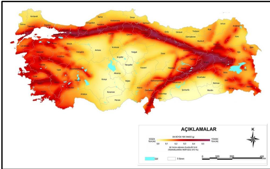
Şekil 3.4: Türkiye Deprem Tehlike Haritası
